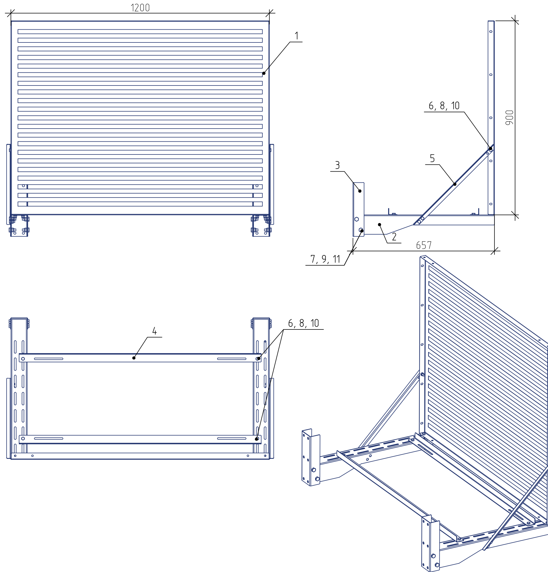
Корзина для кондиционера KORZ.900(h)x1200x600.T3
